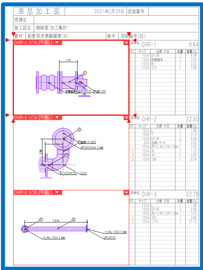
単品加工図(3段)
